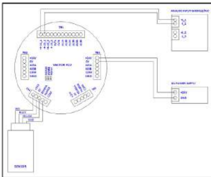
Рисунок 4-10: Проводка Vector для модуля аналогового ввода с токовыми входами и одним преобразователем ПГУ-903У
