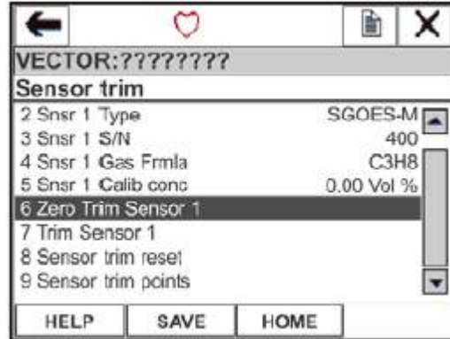
Рисунок 5-12: Экран подстройки преобразователя ПГУ-903У (Нуль)
