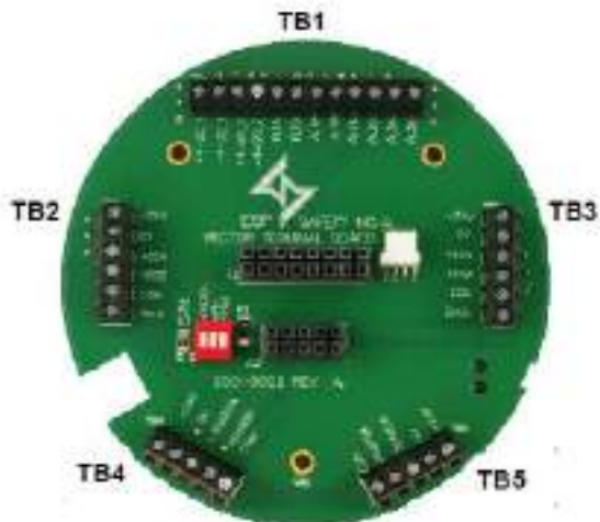
Рисунок 4-9: Клеммная колодка
